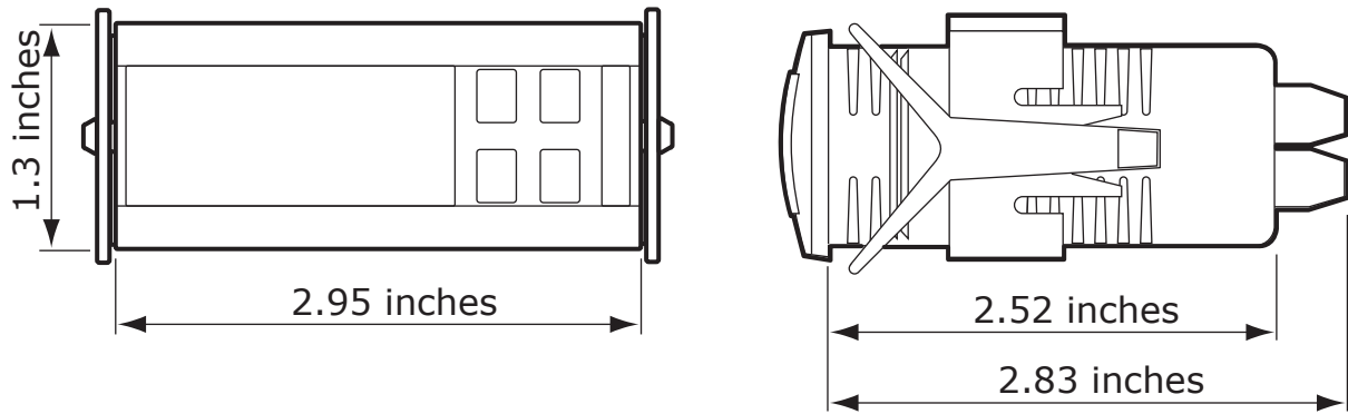
IR32W*
